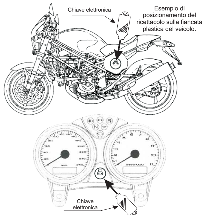
Esempio di posizionamento del ricettacolo su cruscotto del veicolo.
