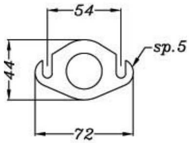
Vista da "A" Flangia "99A"
