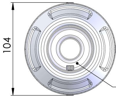
dB-killer Ø22 Cod.303430803
