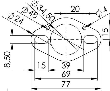
"S.S. flange" Cod.206443
